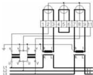
trifase 3 fili 2 TA + 2 TV
